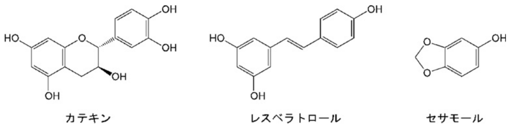
Fig. 5 フェノール性水酸基を有する天然抗酸化物質
