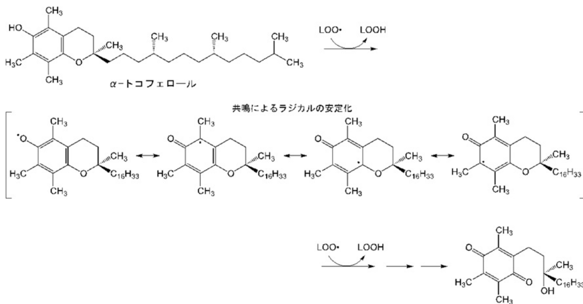
Fig. 4 α-トコフェロール (ビタミンE) の抗酸化機構
